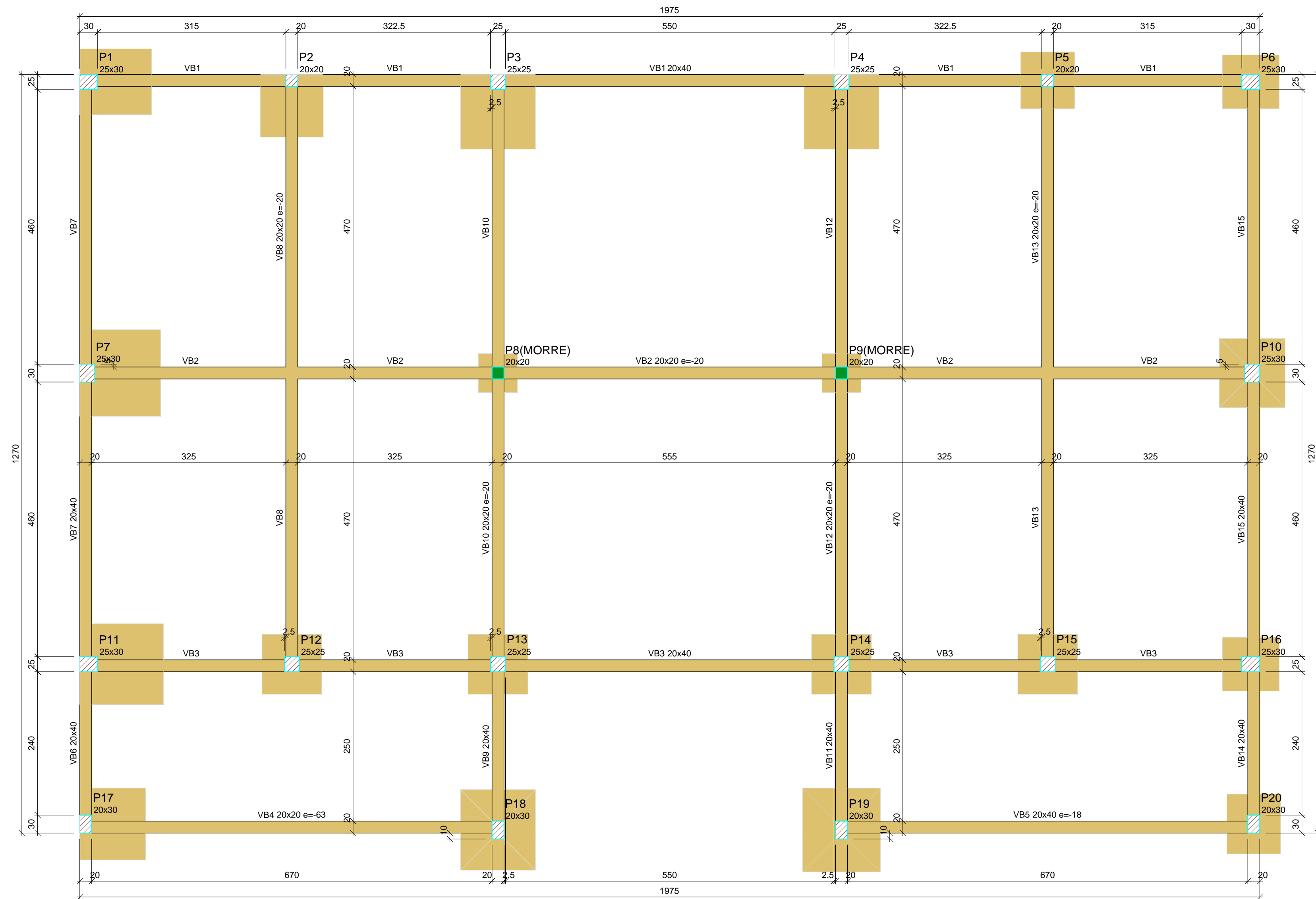
Forma do pavimento Baldrame escala 1:50
