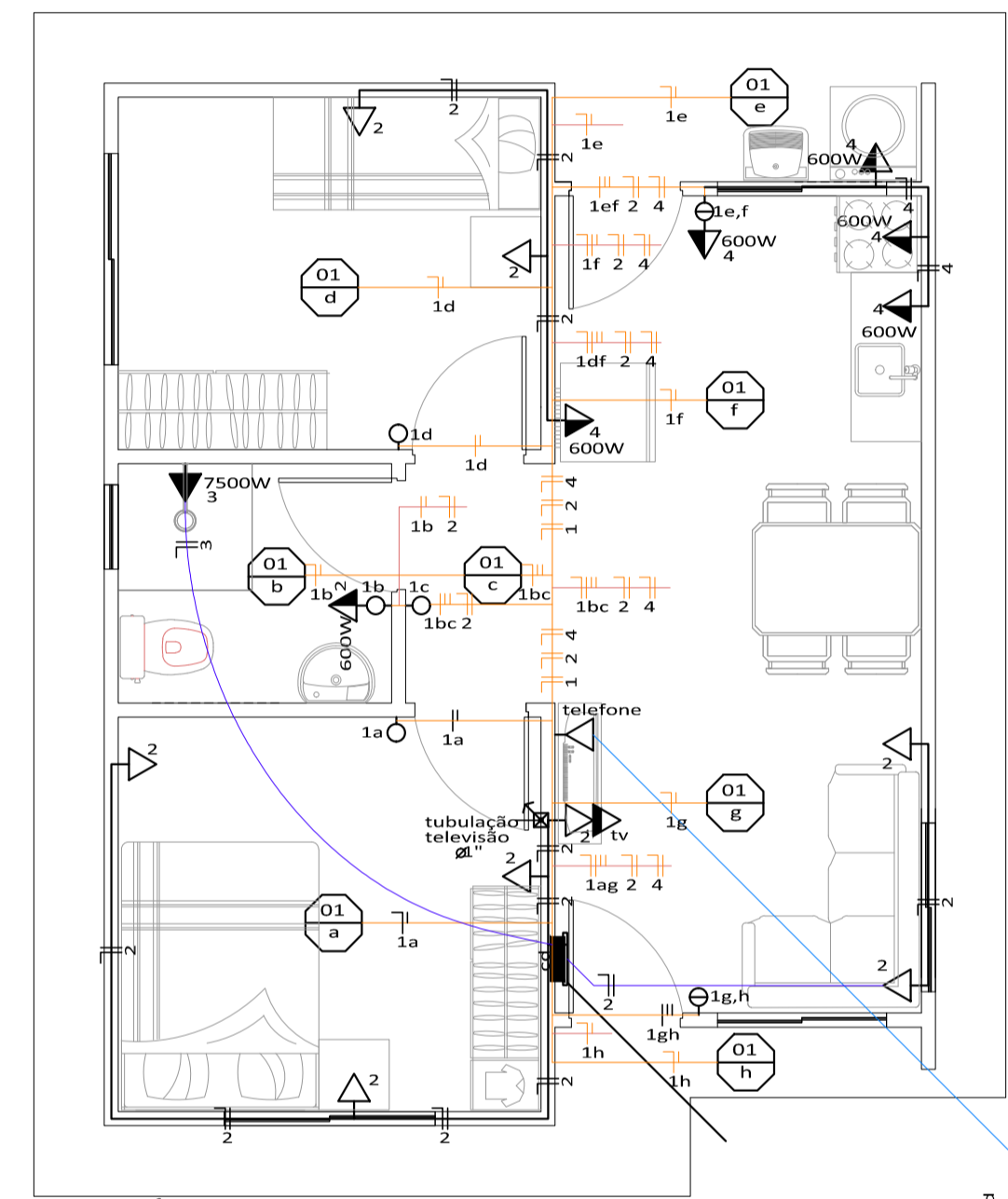
ELÉTRICO Escala 1/50
