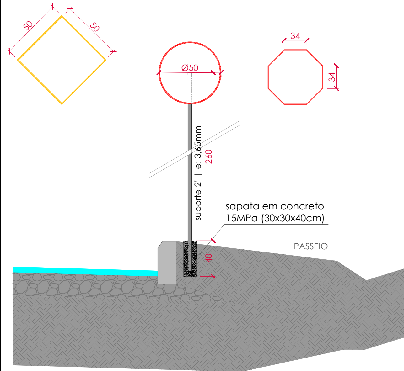
DETALHE PLACAS sem escala
